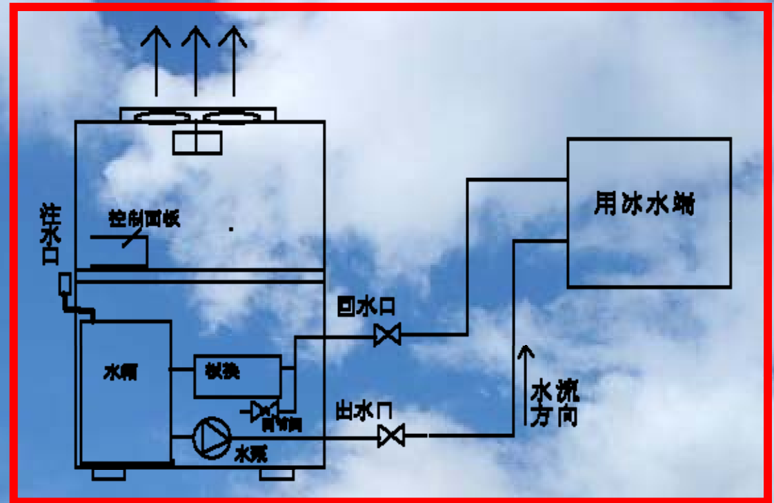
冰水系统图
